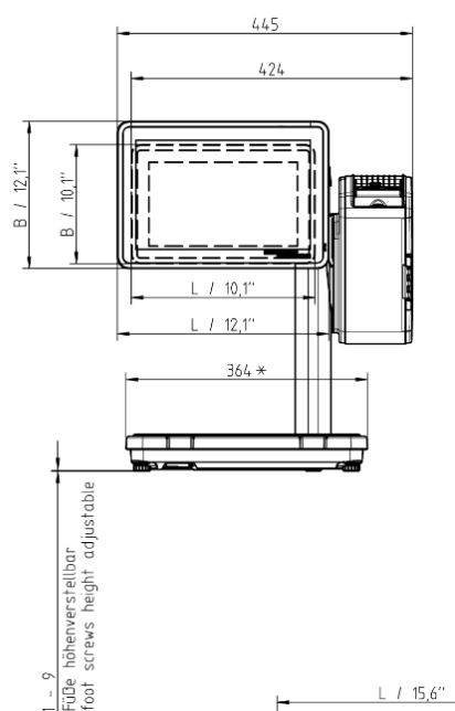
Q1_expert_800_front_view_01
