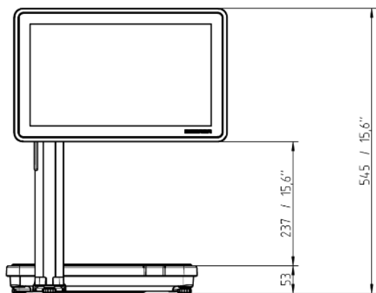
Q1_expert_800_display_view_01
