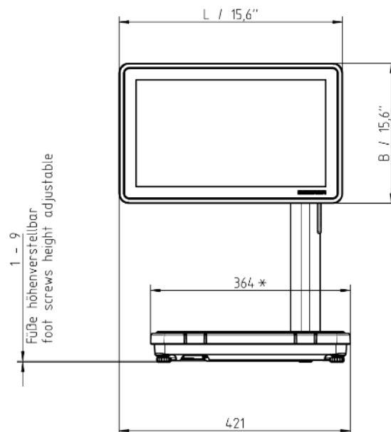
Q1_expert_800_display_view_02
