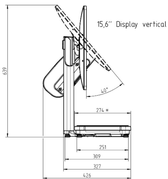
Q1_expert_800_side_view_15,6_display_vertical
