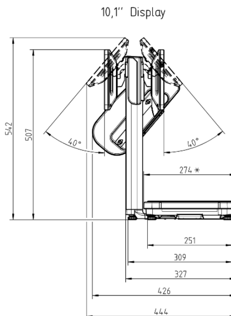
Q1_expert_800_side_view_10,1_display
