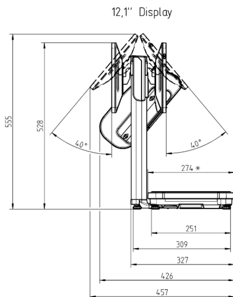
Q1_expert_800_side_view_12,1_display
