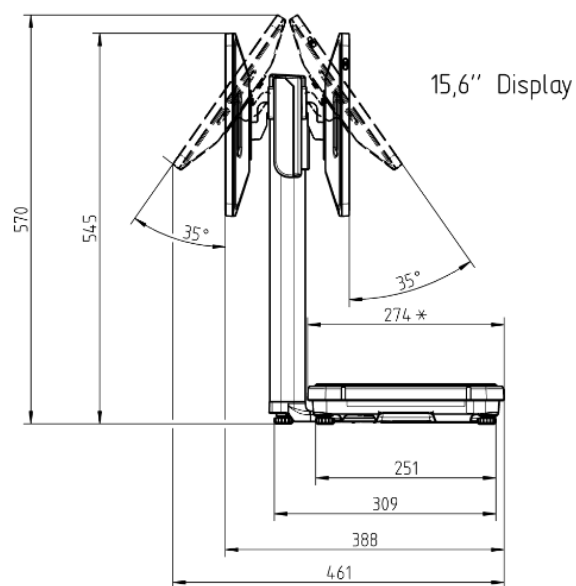
Q1_expert_800_side_view_15,6_display
